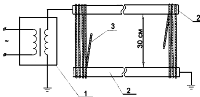
Рис.2.4. Схема электрических испытаний изолирующего каната:
